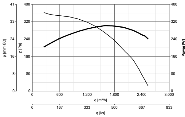
VORT QBK SAL-KC EVO 315 T4 0.25kW code 43153
