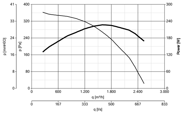
VORT QBK SAL-KC EVO 355 T4 0.25kW code 43155
