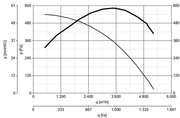
VORT QBK SAL-KC EVO 500 T4 1.5kW code 43159
